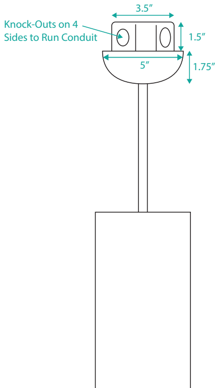
J-Box Options
